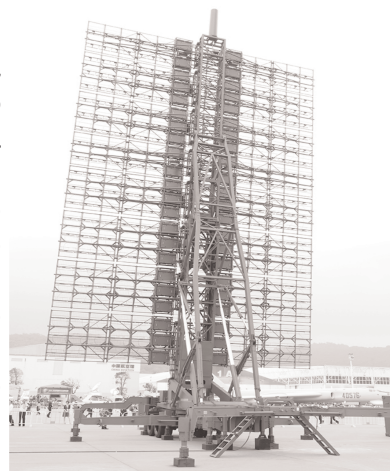
Εικόνα 4: Το ραντάρ CETC JY-27A Skywatch-V, το πρώτο κινεζικό ραντάρ VHF AESA, στην έκθεση αεροναυτικού υλικού Zhuhai στην Κίνα, το Νοέμβριο 2014 ( http://aviationweek.com/technology/new-radars-irst-strengthen
