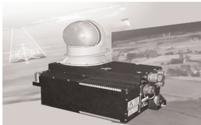
Εικόνα 9: Το σύστημα Skyward G-IRST (Infra-Red Search & Track) του Α/Φ Gripen NG, ένα από τα πιο εξελιγμένα συστήματα σήμερα, της Finmeccanica – Selex ES ( http://www.leonardocompany.com/en/-/skyward-g-irst )
