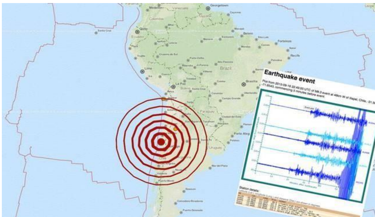
Εικόνα 33: Επίκεντρο Σεισμού στη Χιλή (Πηγή:
