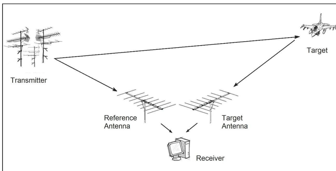
Εικόνα 7: Τα παθητικά ραντάρ (PCL) βασίζονται στην σύγκριση του σήματος που λαμβάνεται από έναν υφιστάμενο σταθμό FM, TV, GSM κλπ, και ανάλογο σήματος μέσω ανάκλασης από τον στόχο. Το δεύτερο σήμα αποτελεί “αντίγραφο” του πρώτου, σε πολύ χαμηλότερη στάθμη, με μία χρονική καθυστέρηση και με μία μετατόπιση στο φάσμα της συχνότητας ( https://www.researchgate.net/publication/306372794_Parousiase_-_Exetase_Ylopoieses_Pathetikou_Rantar_PASSIVE_RADAR ).
