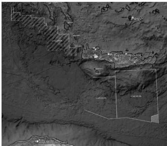
Σχήμα 2α: Το αρχικό της CHEVRON (με κίτινη διαγράμμιση) καθώς και τα δύο νέα νότια της Κρήτης
