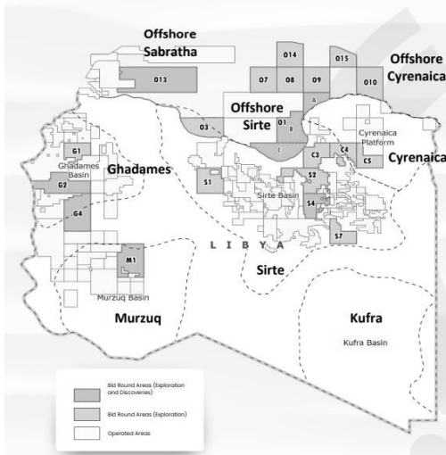
Σχήμα 3: Νέος γύρος παραχωρήσεων για έρευνα υδρογονανθράκων της Λιβύης σε 22 περιοχές
